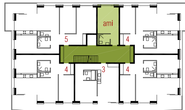
5ème étage
