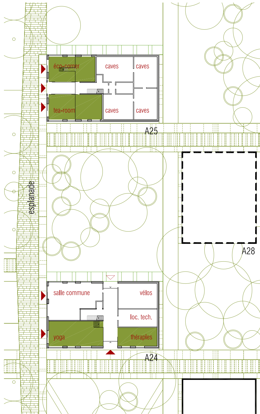
rez inférieur
