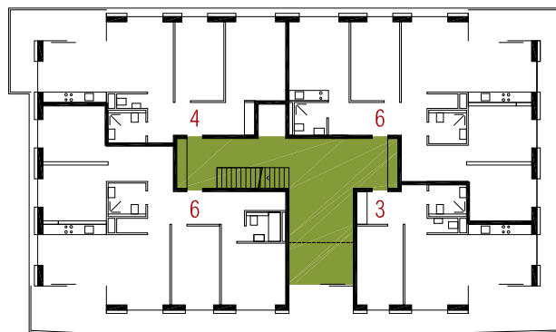
2ème étage
